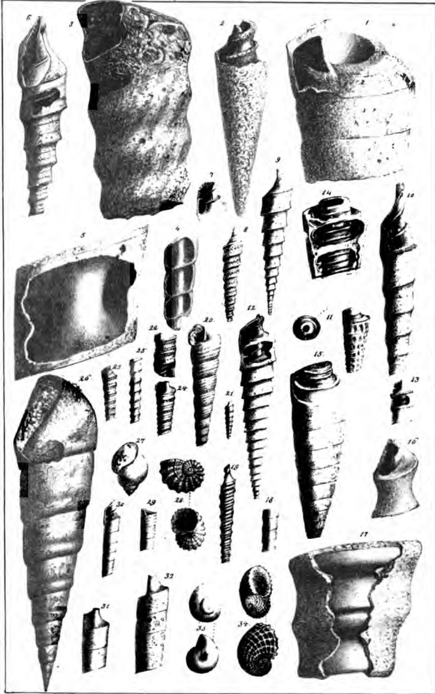
Rosenfeldt, Java.
